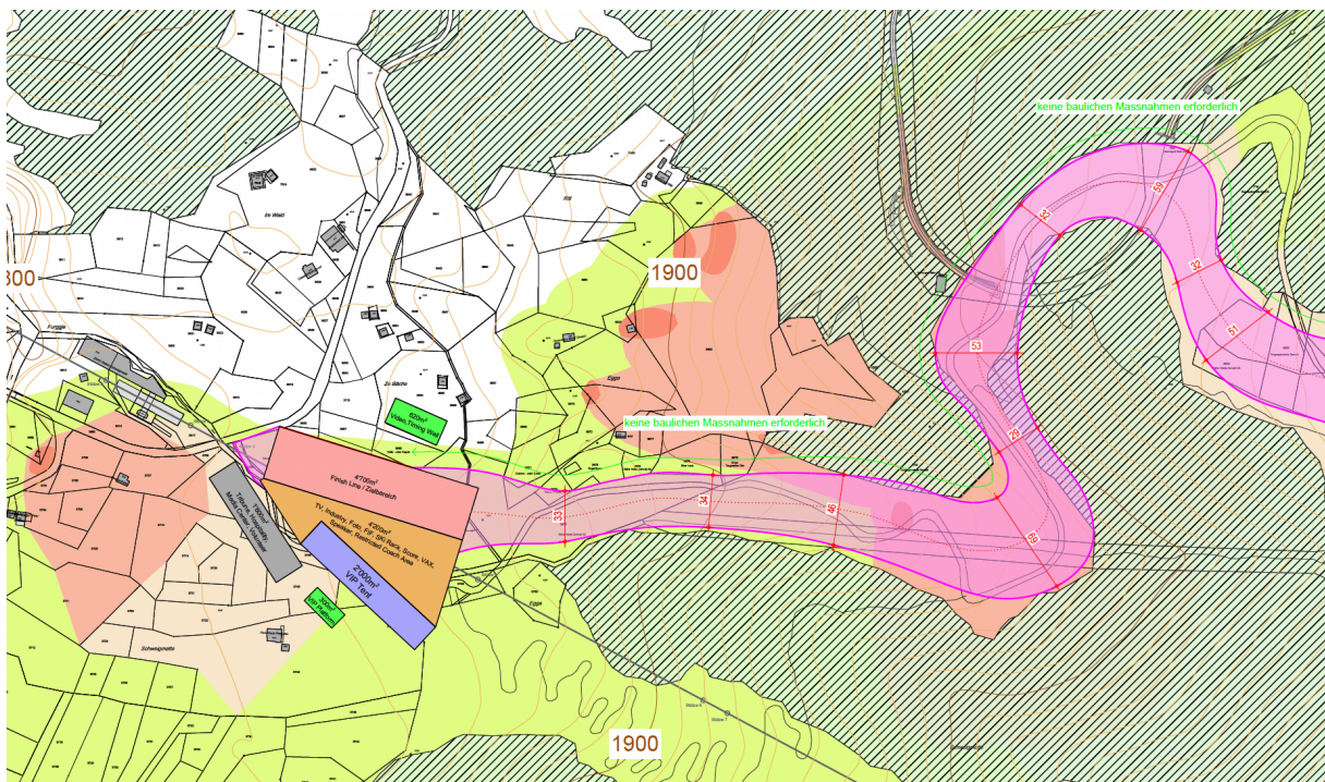
Abb. 17: Ausschnitt Situationsplan 1:2'000 Auflageprojekt (LABAG Bauingenieure AG) Sektor Hubelti / Unerri Riffelalpa – Schweigmatten
