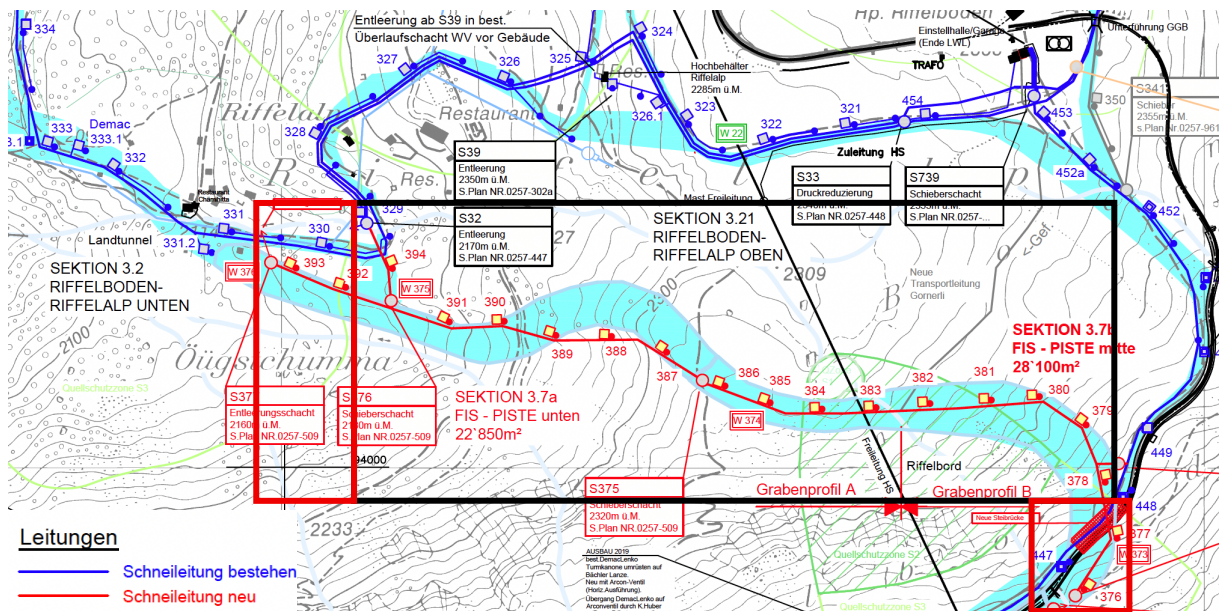
Abb. 14: Planausschnitt Entwurf Situationsplan 1:5'000 (Brigger + Käch Bauingenieure AG) geplante Anpassung des Beschneisystems im Sektor Galerie Riffelbord – Hubelti / Chämihitta mit Übersicht bereits bewilligte Schneeanlage (schwarze Umrandung) und projektspezifische Anpassung neu (rote Umrandung)
