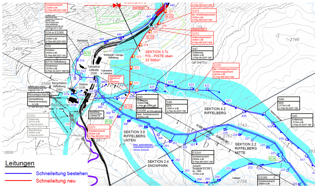
Abb. 10: Planausschnitt Situationsplan 1:5'000 (Brigger + Käch Bauingenieure AG) mit geplanter Anpassung des Beschneigungssystems im Sektor Sektor Gifftitli – Galerie Riffelbord
